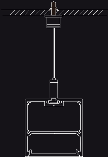
PENDANT 悬挂式
