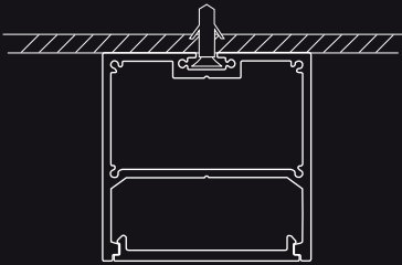
SURFACE MOUNTED 固定式
